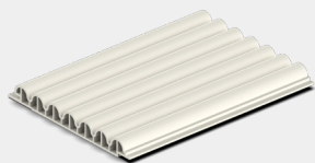
SPSQ-527 (แผ่นสำเร็จ / ฟิล์มลามิเนต) Size : 18 x 157 x 2900 mm.
